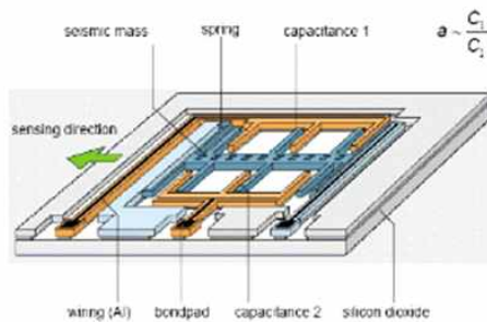
&lt;MEMS chip 작동원리 다이어그램(3축 가속도 센서)&gt;
