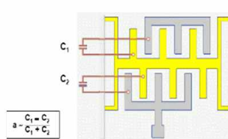
&lt;MEMS chip 작동원리 다이어그램(3축 가속도 센서)&gt;
