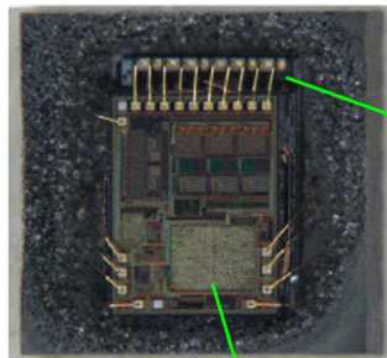
상단 칩(ASIC IC)
